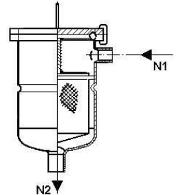
Siebkorbfilter – Beutelfilter leichte Ausführung Größe 0 - II
